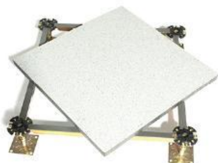
有横梁地板及支架安装
