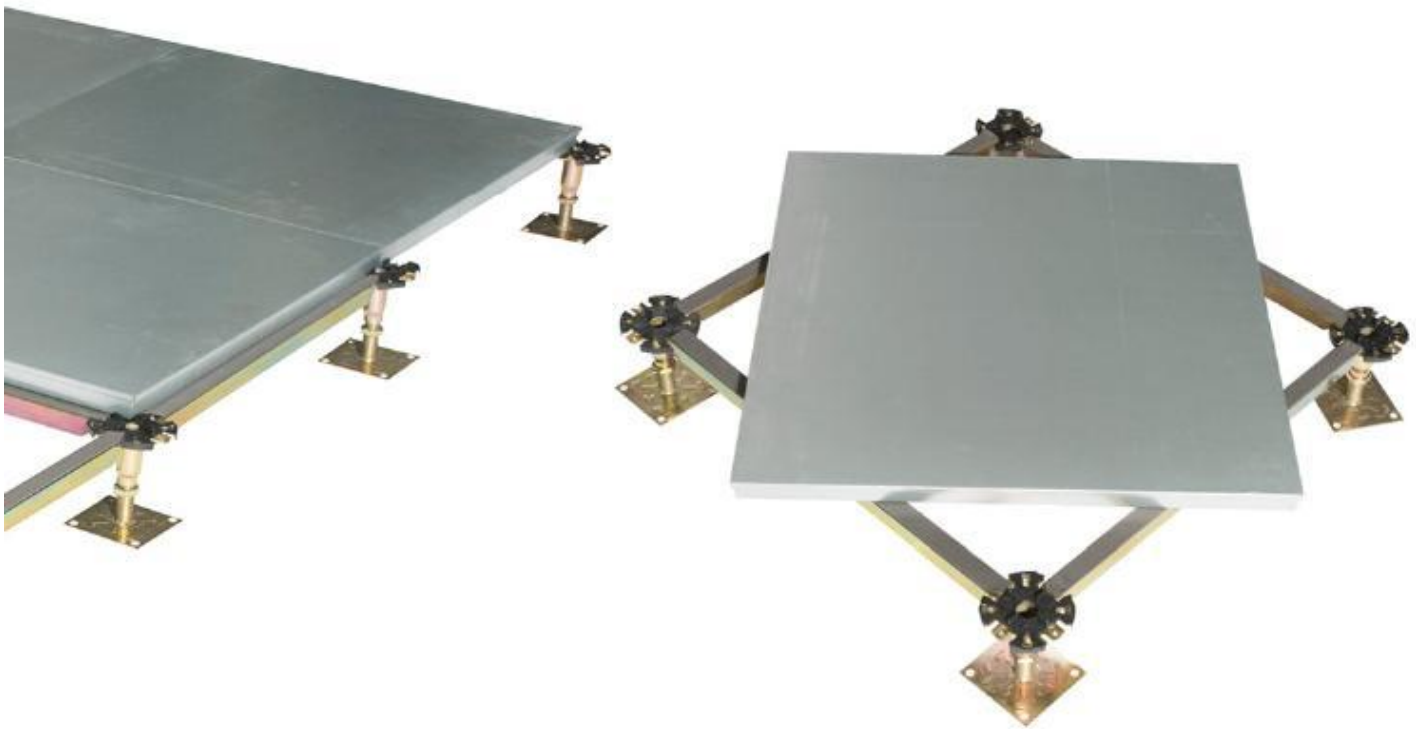
有横梁地板及支架安装
