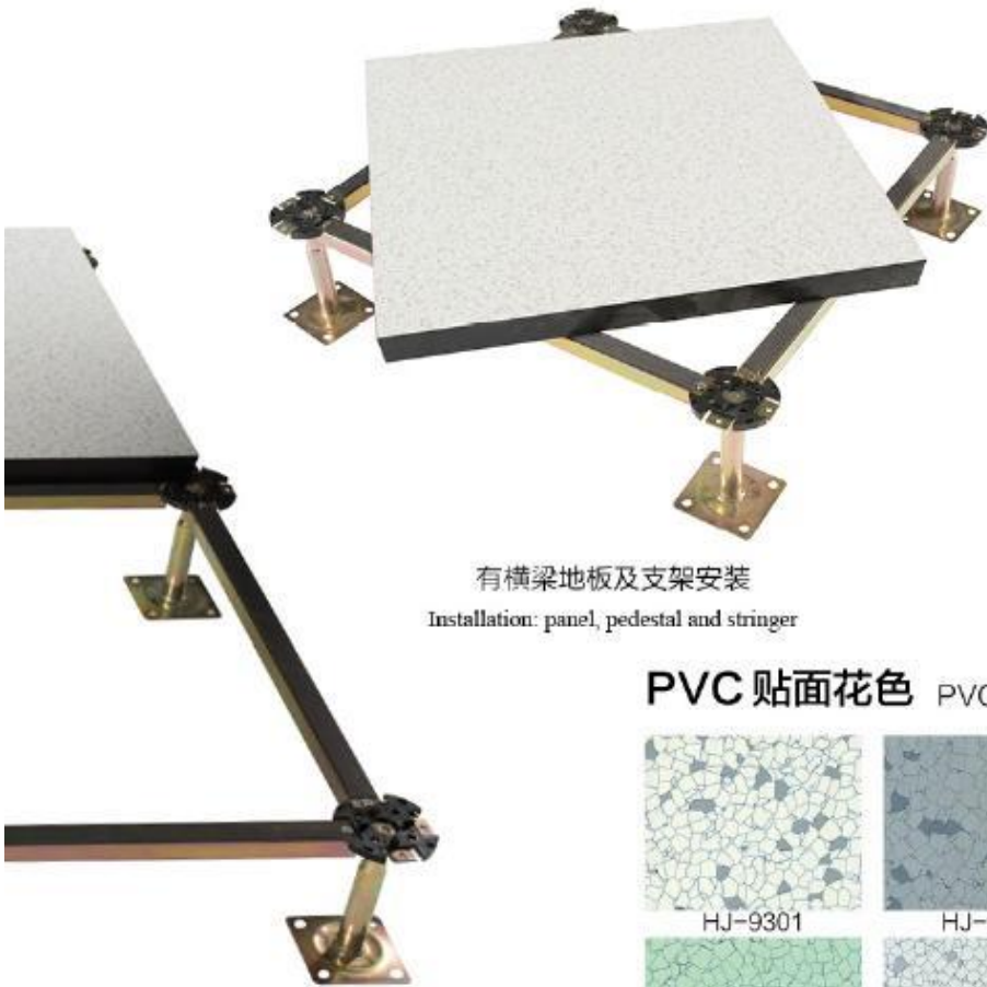
支架: 可调支架高度为 100-500mm pedestal range 100-500mm
